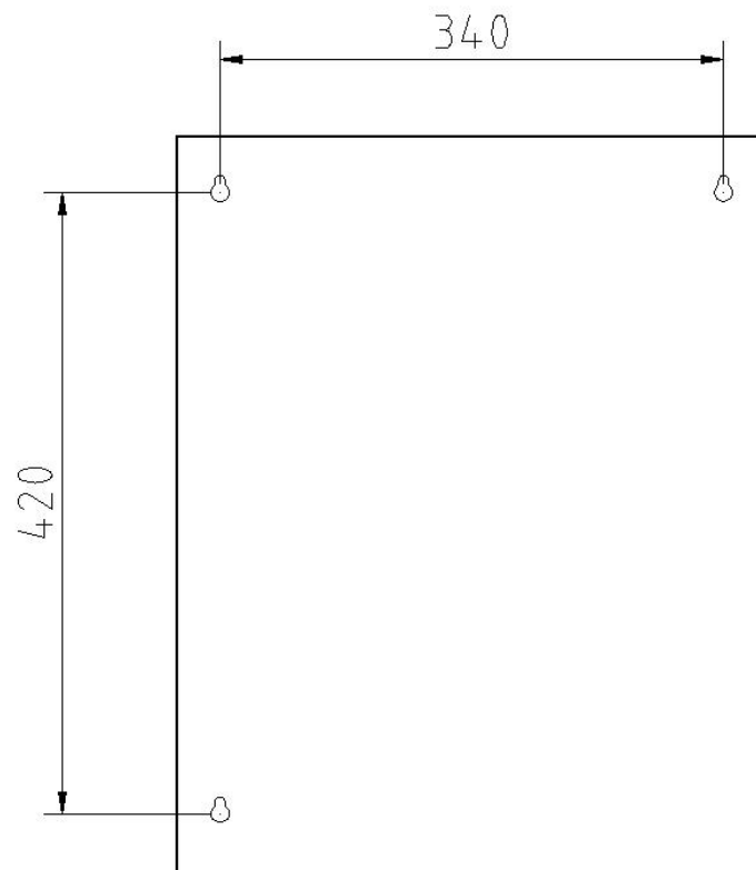
图4 设备安装尺寸图
